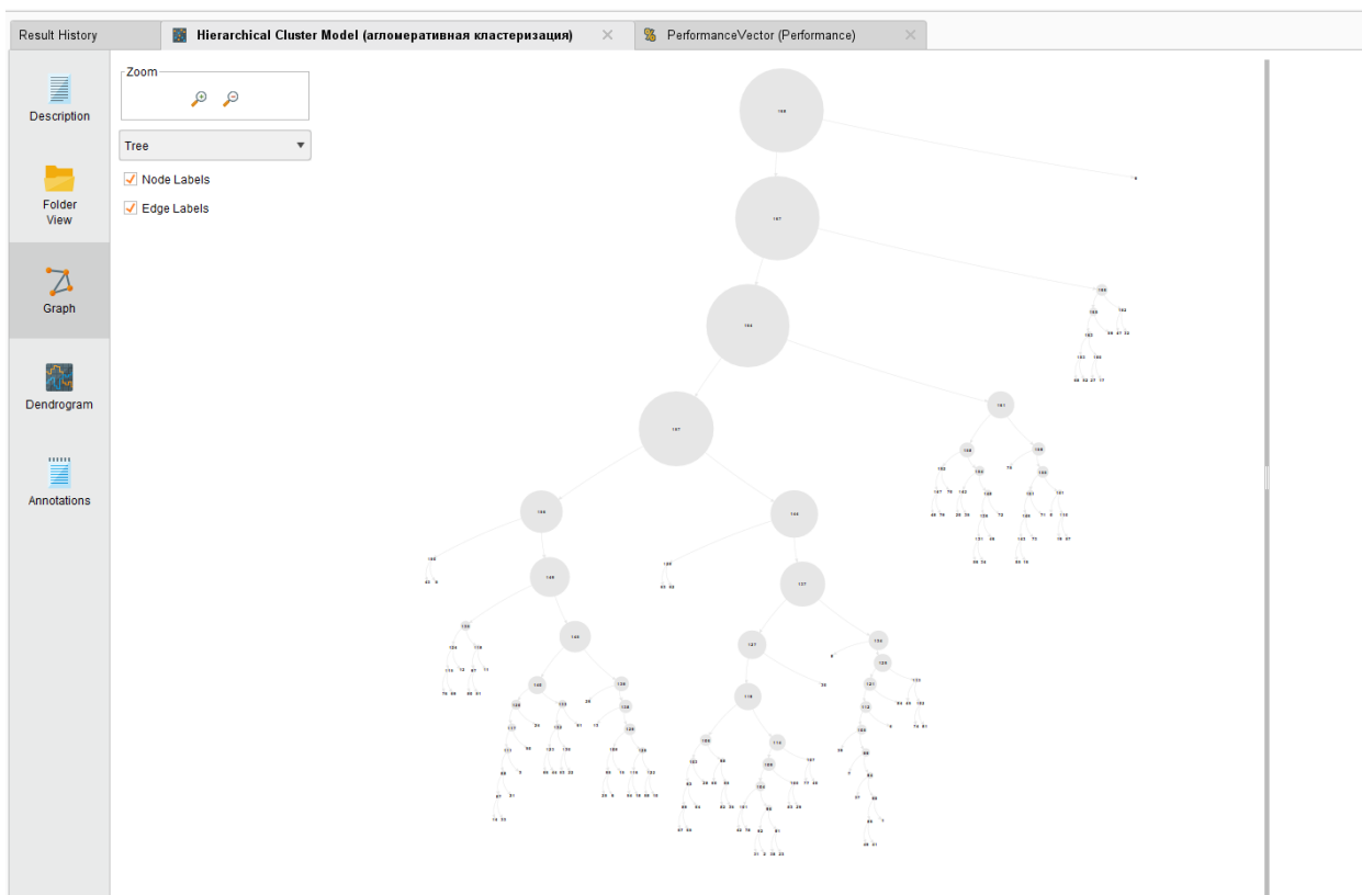
Рисунок 14 – Графы
