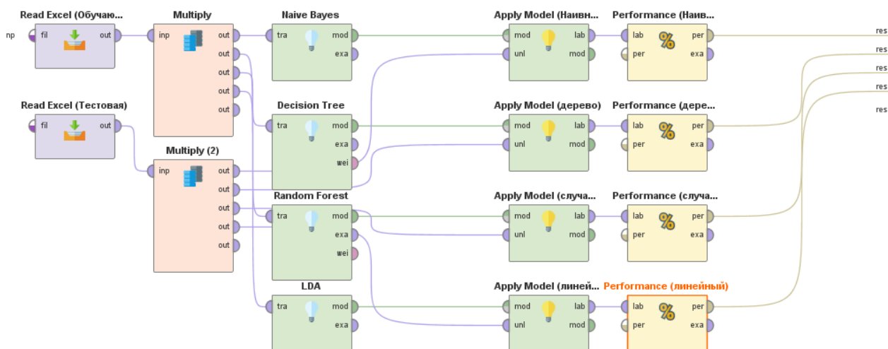
Рисунок 16 - Процесс классификации
