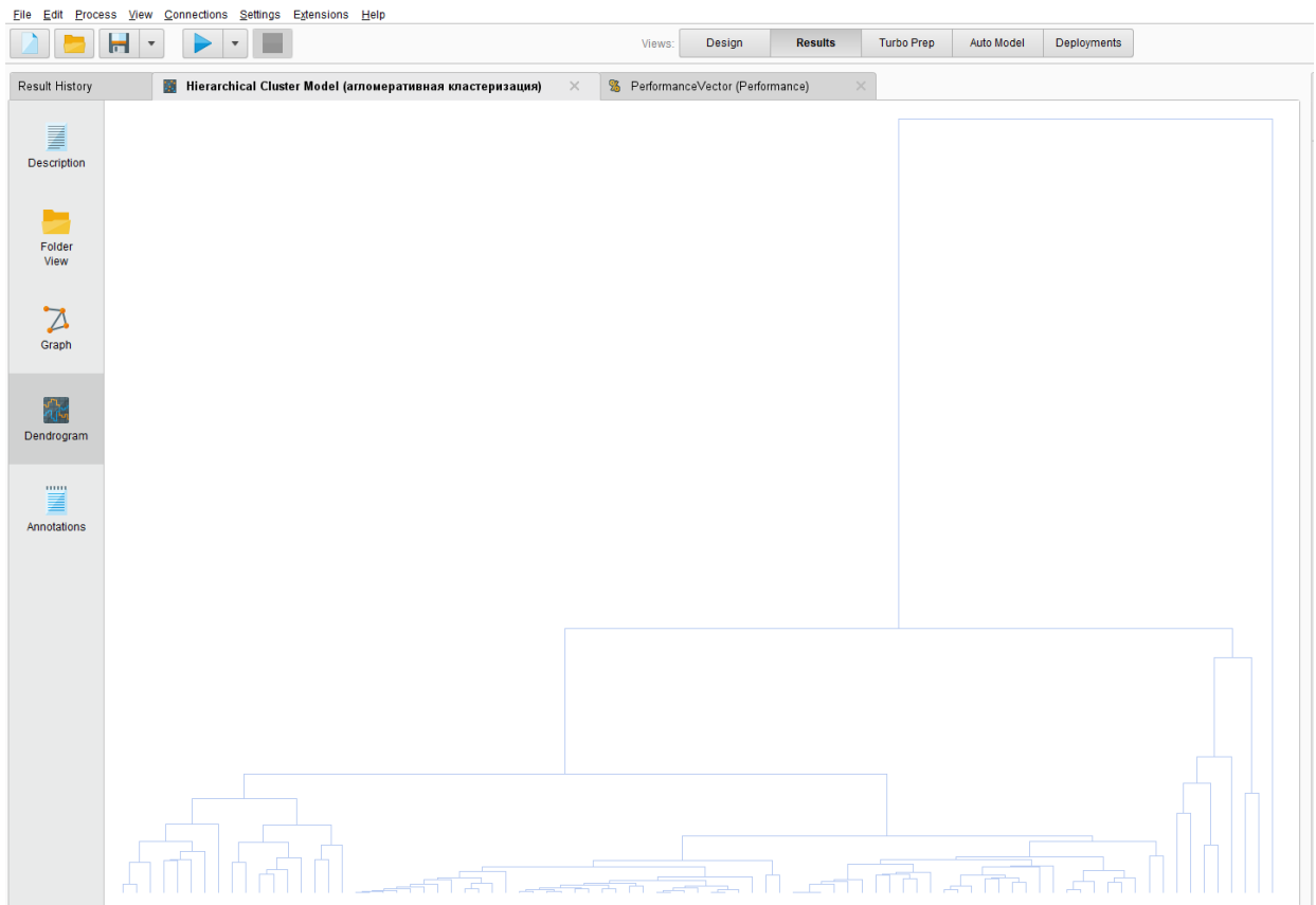
Рисунок 13 - Иерархическое дерево
